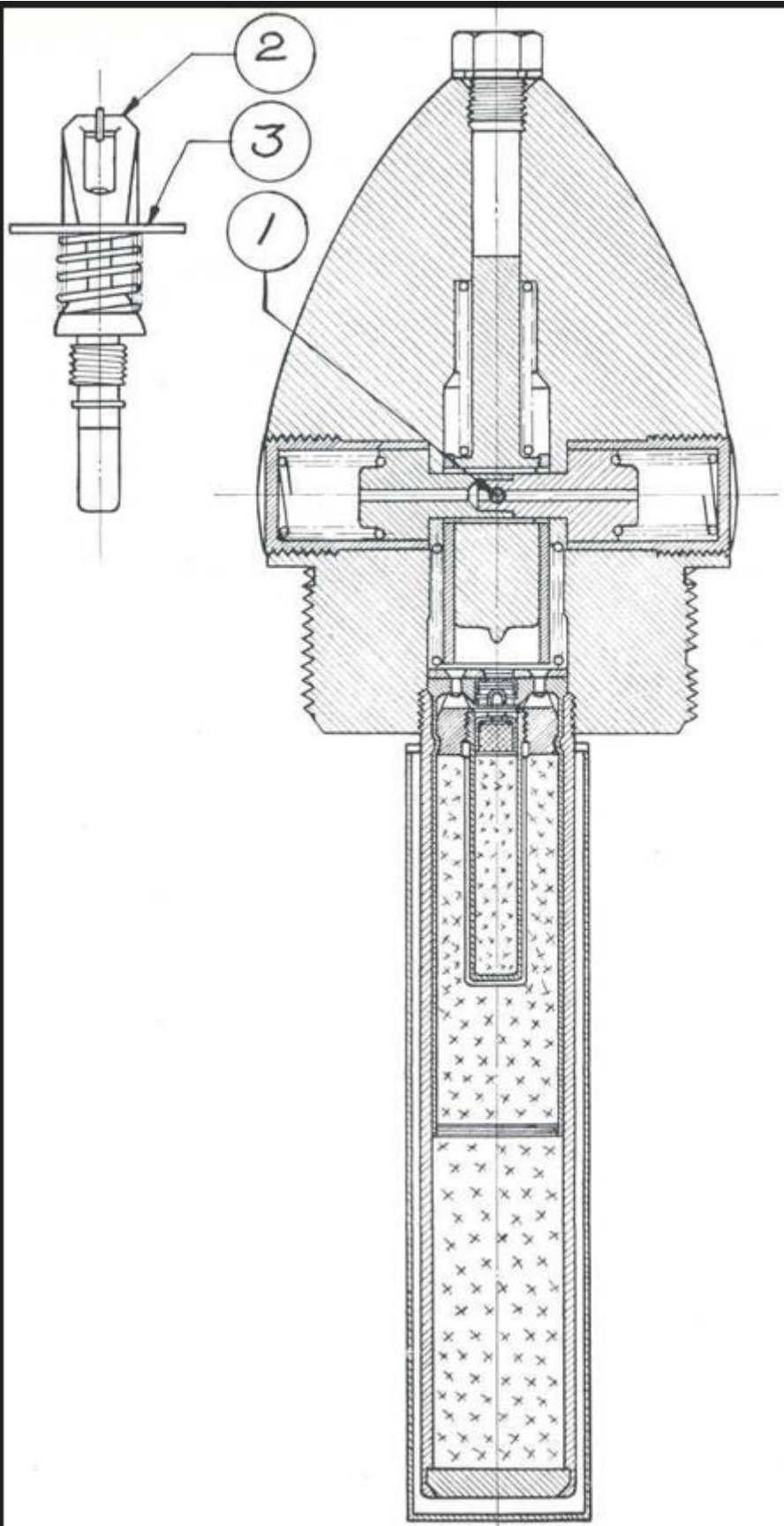
Fig. 10. Spetsrör m/32-37 med detonator.
